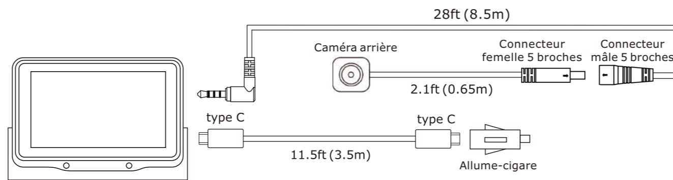
Installation sur le pare-brise
