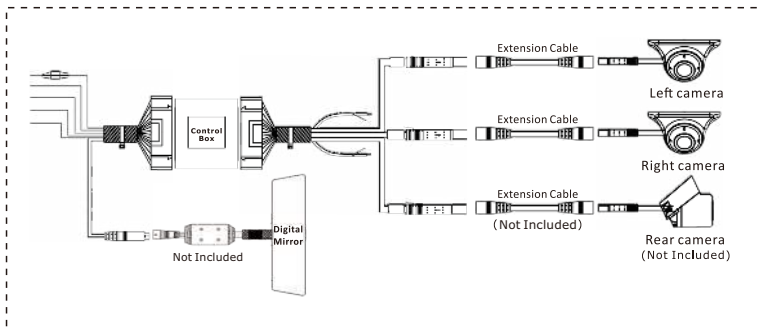
OPTIONAL CM-D700 AHD (AHD VIDEO SWITCHER)
